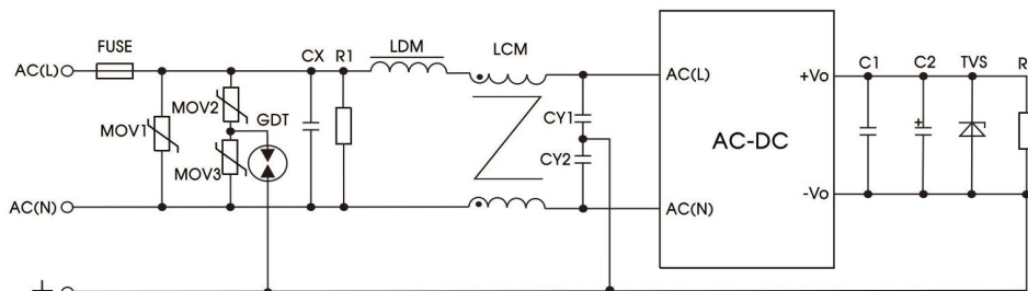
图 2：EMC 更高要求推荐电路
